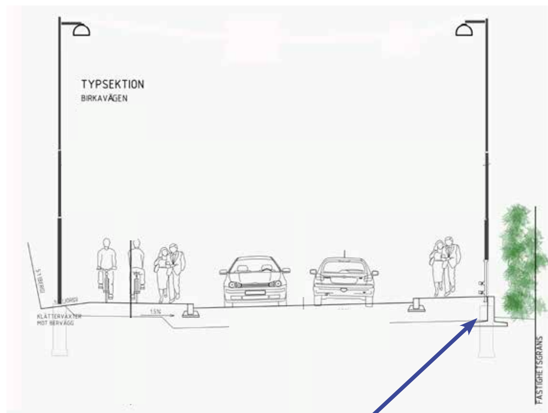
Typsektion för Birkavägen. Sektion är från förstudien gjord 2018 SWECO för Nacka kommun
