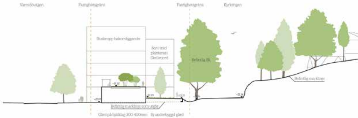
Möte mellan gård, befintliga ekar och Kyrkstigen. Dike och mur fungerar som skyfallsränna. Sektion är från Gestaltungsprogram Järle norr 220323 framtaget av ALM
