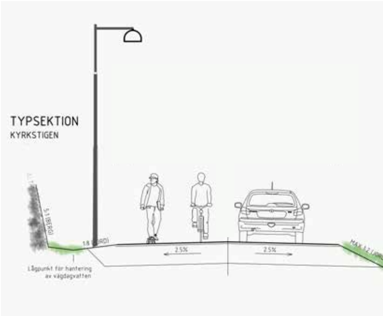
Typsektion för Kyrkstigen. Sektion är från förstudien gjord 2018 SWECO för Nacka kommun
