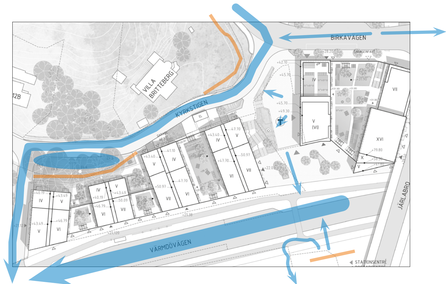
Skyfallets vägen genom Järla Norr området
